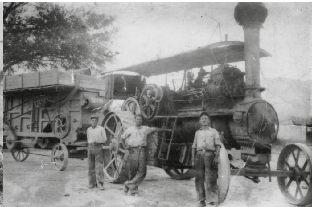
Αλωνιστικό συγκρότημα αποτελούμενο από το ατμοκάζανο με το ψηλό φουγάρο και πίσω την αλωνιστική μηχανή (πατόζα) στο Συκούριο το 1948. Στο μέσον της φωτογραφίας ο μηχανικός Κωνσταντίνος Γκορτσούλης (Γκόλτσος), έχοντας αριστερά τον Ιωάννη Μακρή και δεξιά τον Δημήτριο Γαλλιό.
